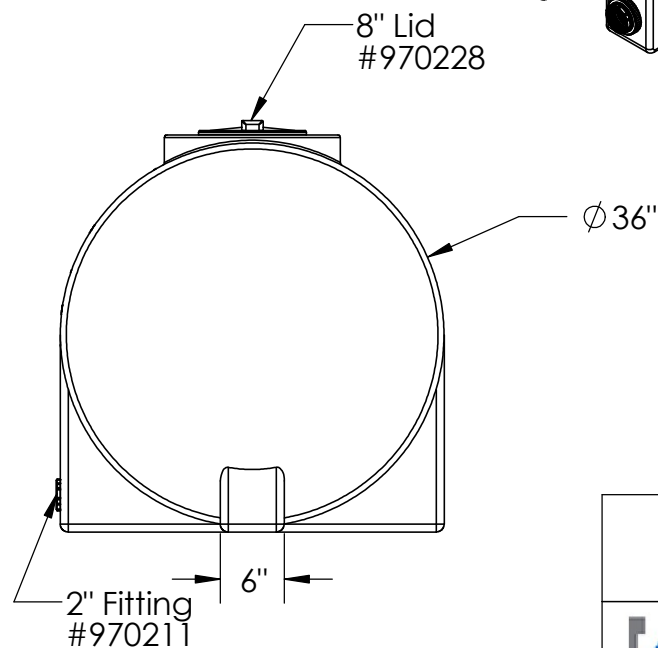
200 Gal Legged Tank
